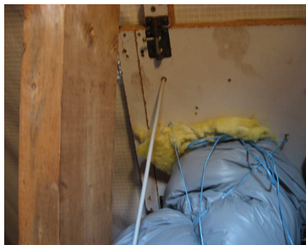
prise d'air d'insufflation montée sur charnières et verrouillée avec des targettes.
